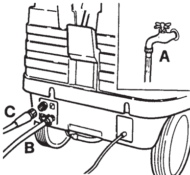
Подключение воды.
