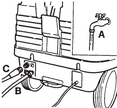
Collegamento idrico.
